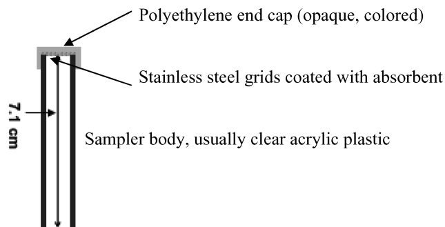
FIG. 1. Diagram of Palmes-type diffusion sampler.
